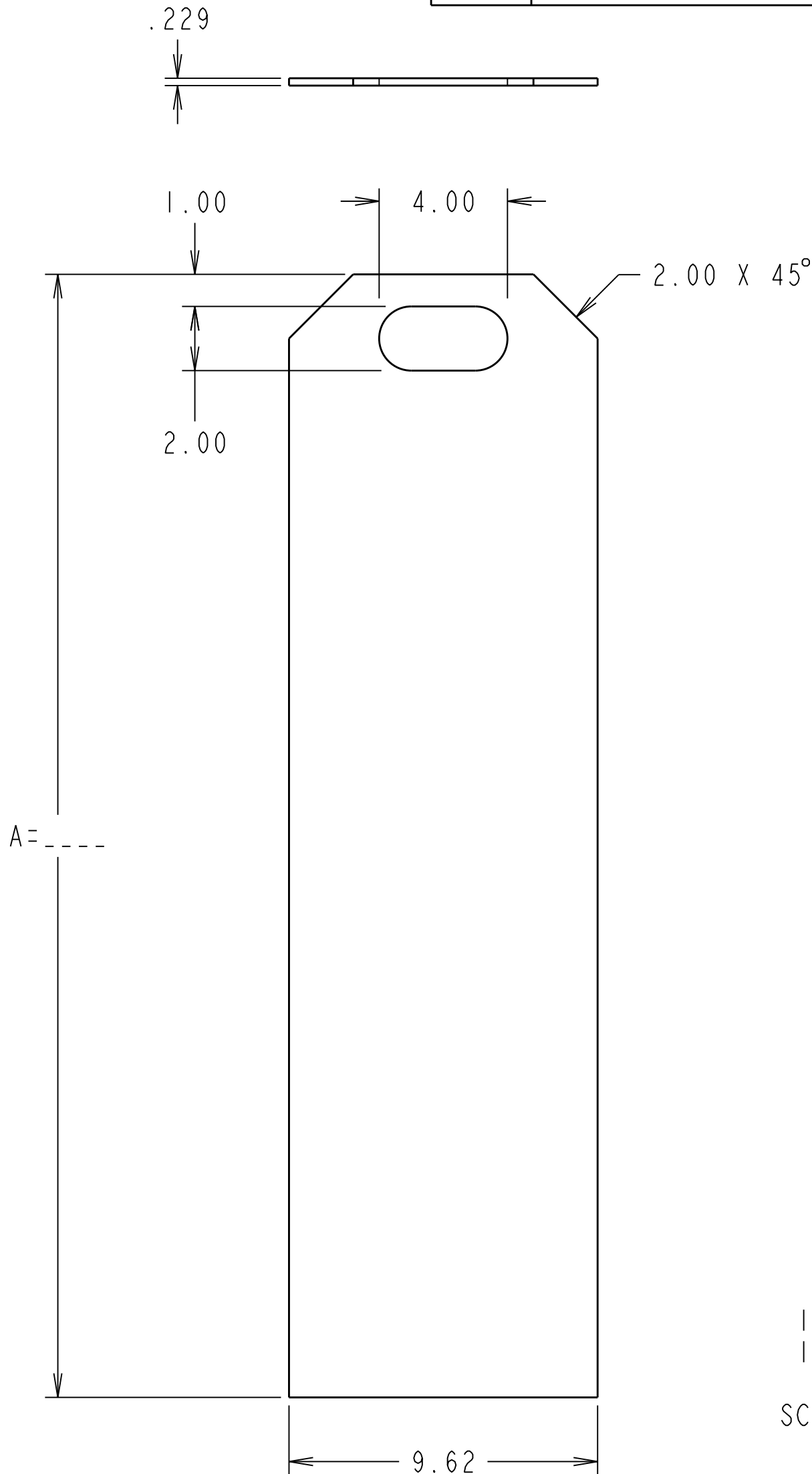
ITEM 20 120-055 2 REQ SCALE 1/4
